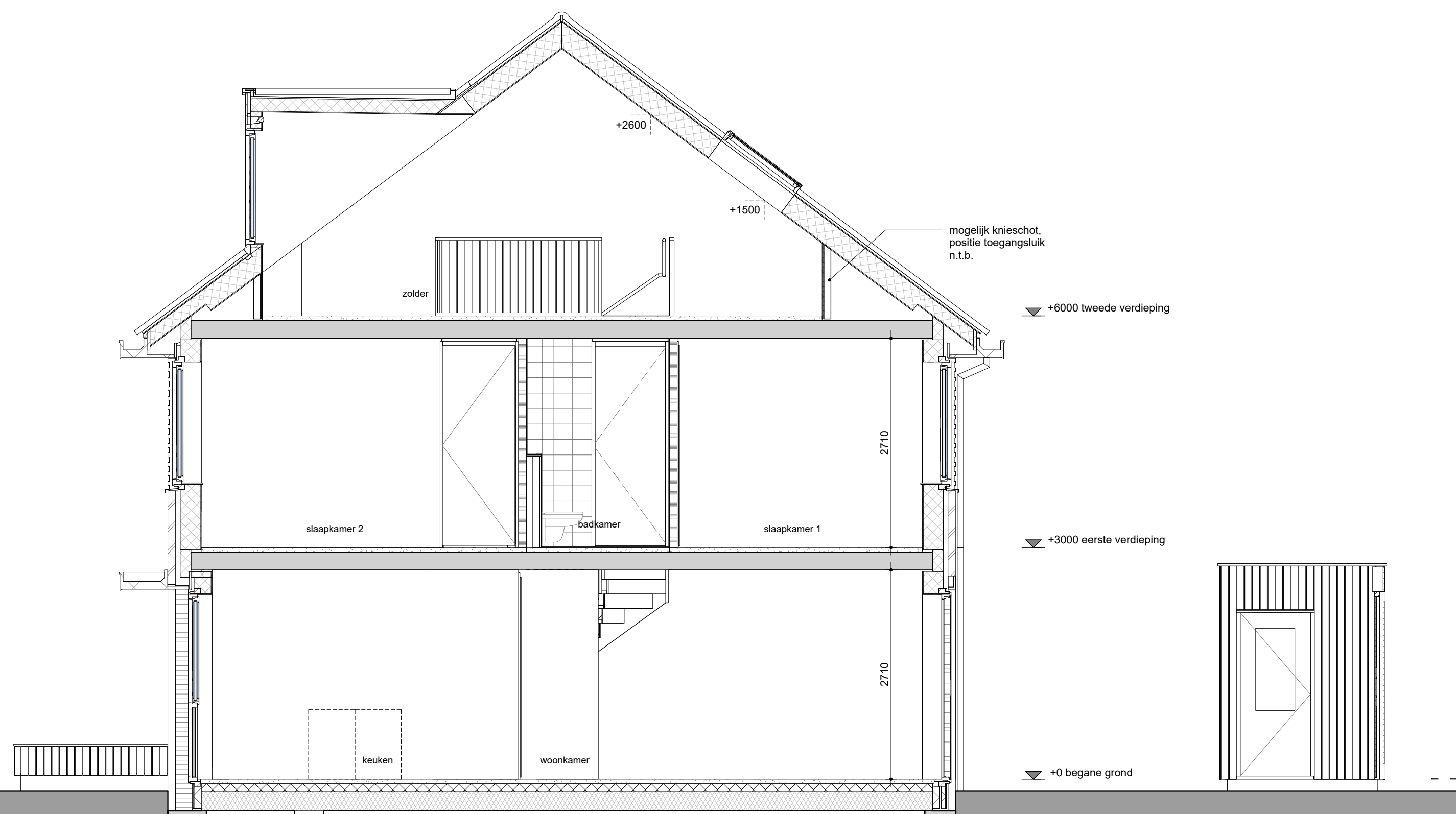
Doorsnede woningtypes B
